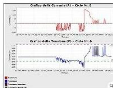
Grafico della tensione di lavoro e della corrente di carica
